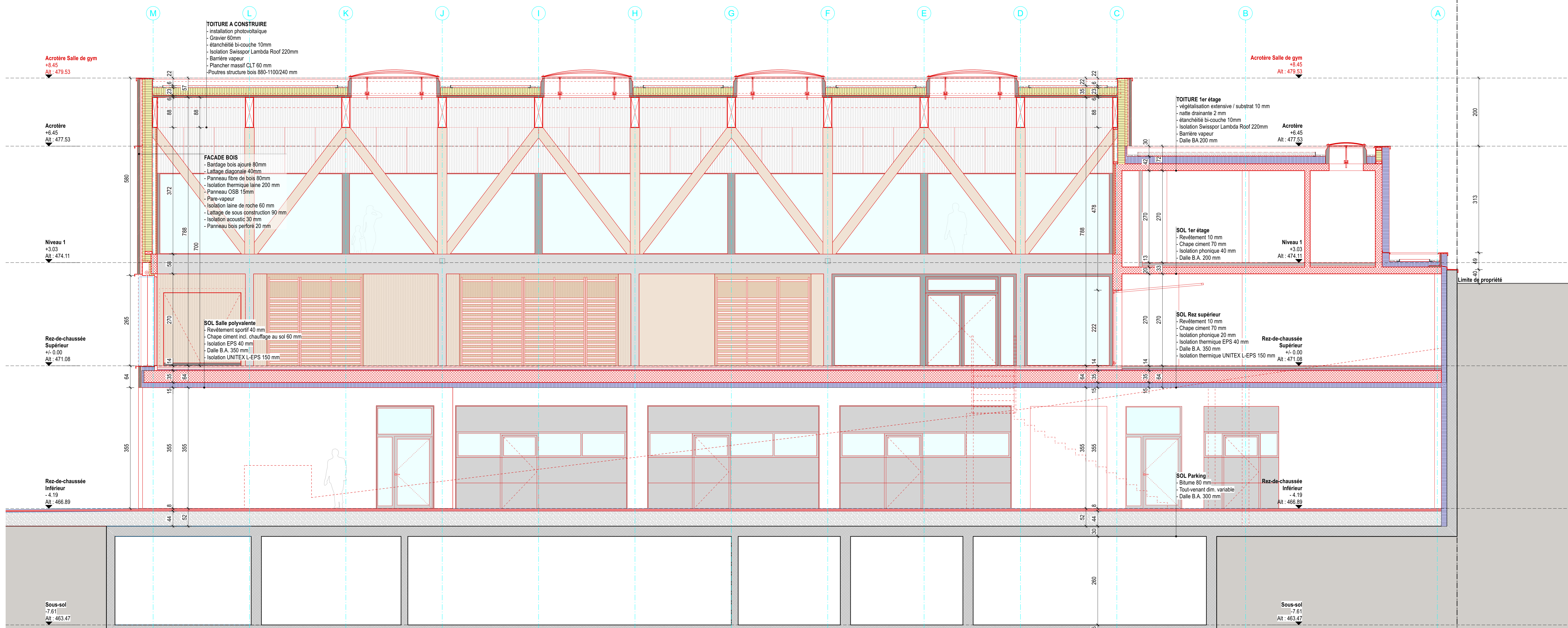
Coupe A
