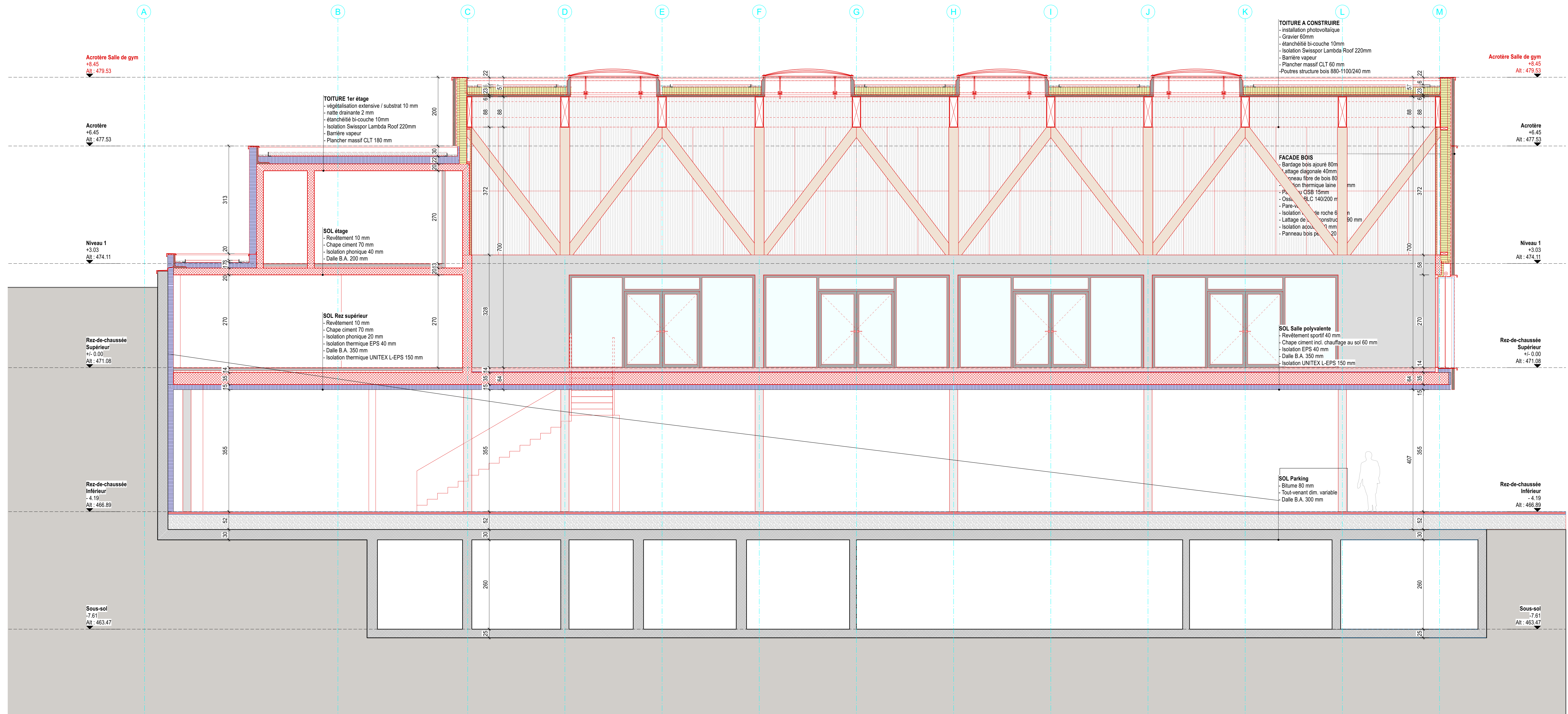
Coupe D
